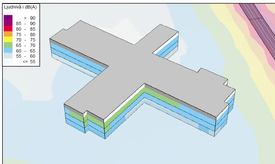
Figur 7. Maximal ljudnivå vid fasad, placeringsvariant 1. Vy från norr. Motsvarar bilaga 2.
