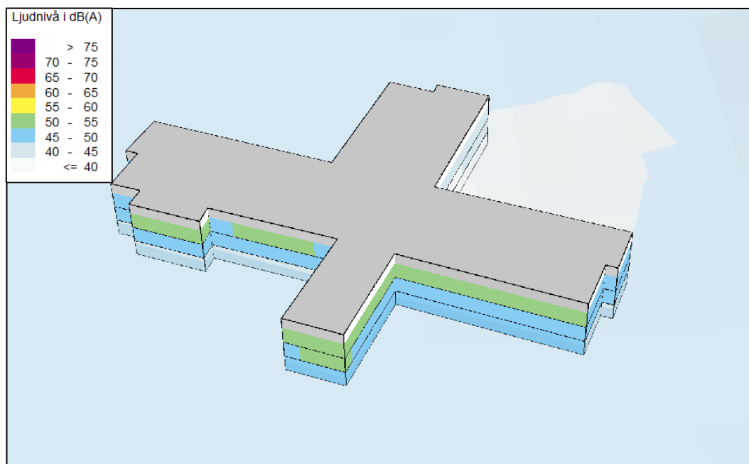
Figur 4. Ekvivalent ljudnivå vid fasad, placeringsvariant 1. Vy från söder. Motsvarar bilaga 1.
