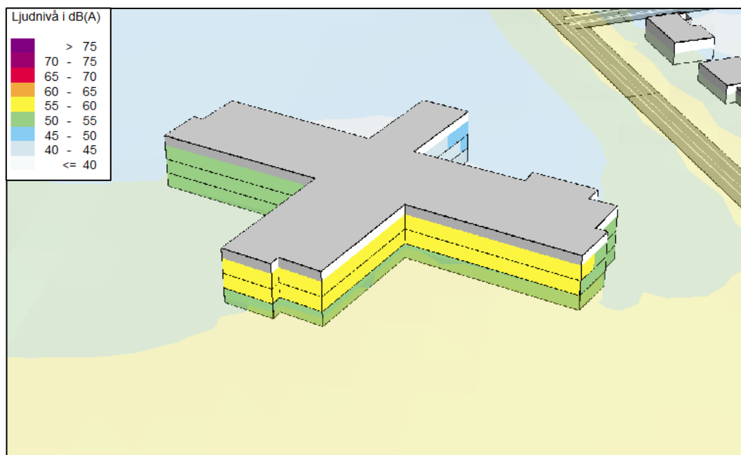
Figur 6. Ekvivalent ljudnivå vid fasad, placeringsvariant 1. Vy från norr. Motsvarar bilaga 1.
