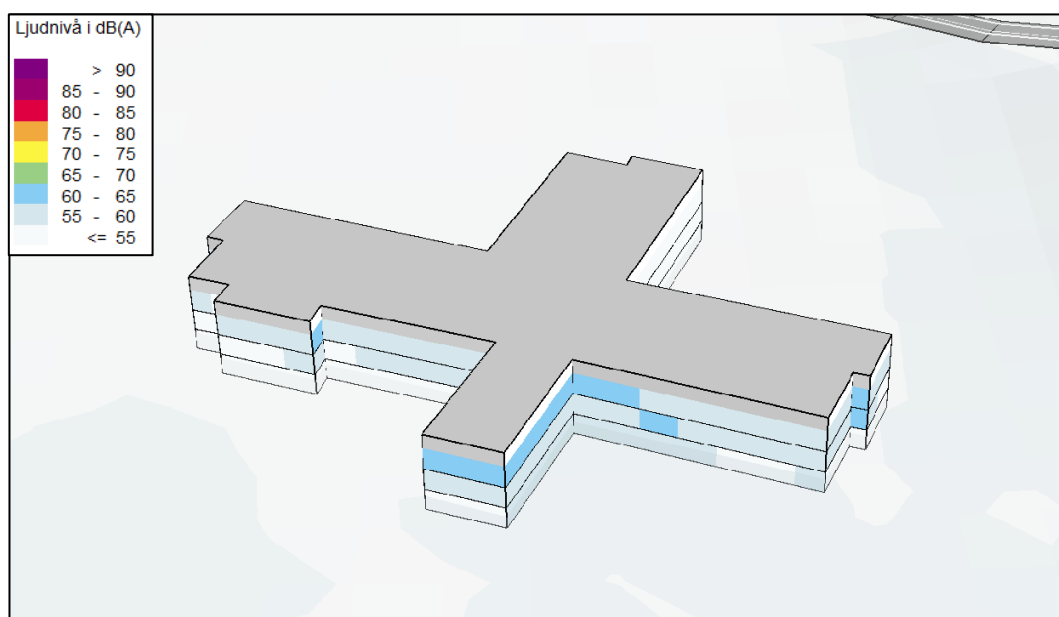
Figur 5. Maximal ljudnivå vid fasad, placeringsvariant 1. Vy från söder. Motsvarar bilaga 2.
